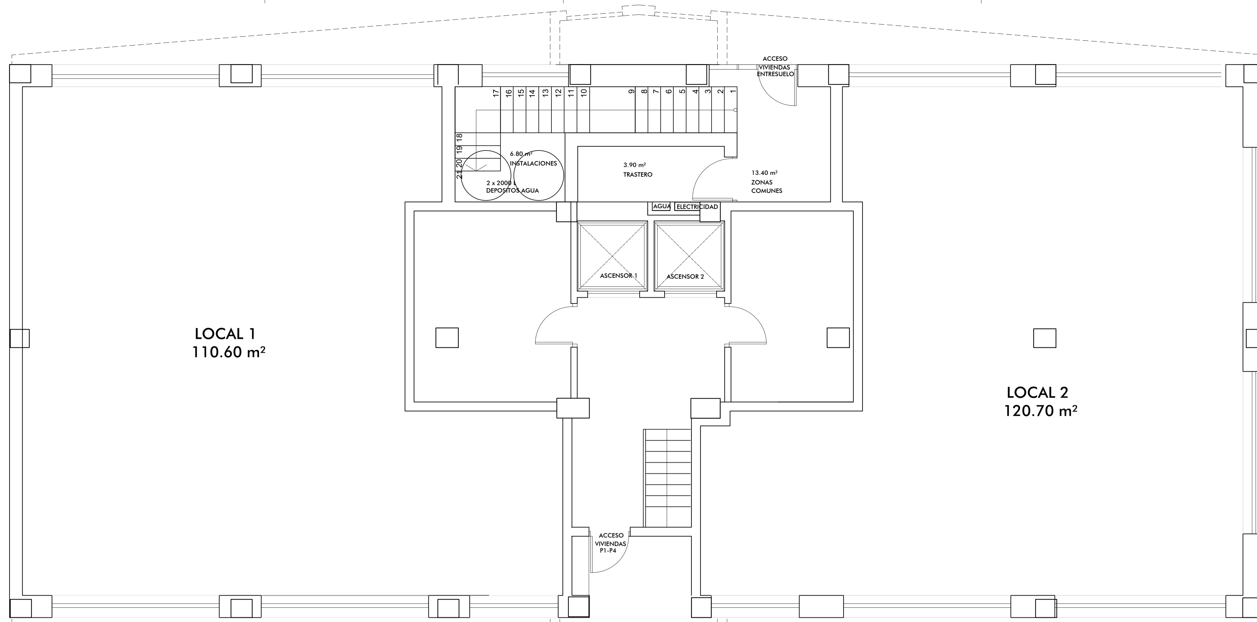
PLANTA BAJA ESTADO REFORMADO (1/50)
