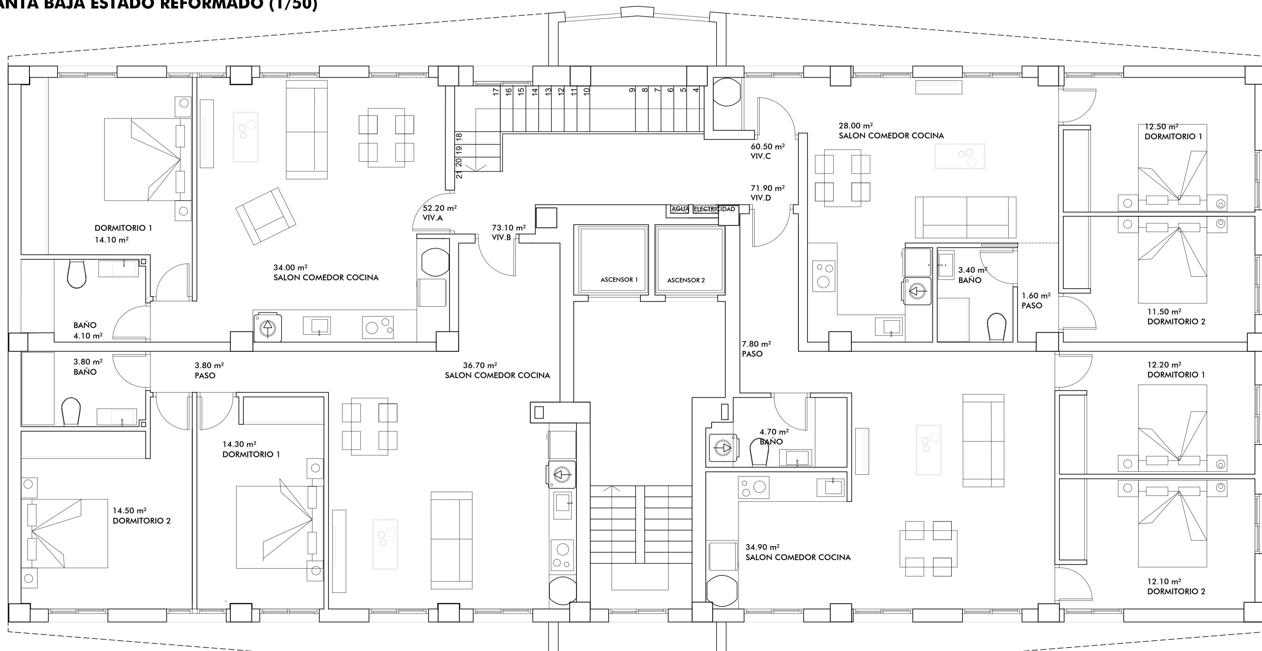
PLANTA ENTRESUELO ESTADO REFORMADO (1/50)
